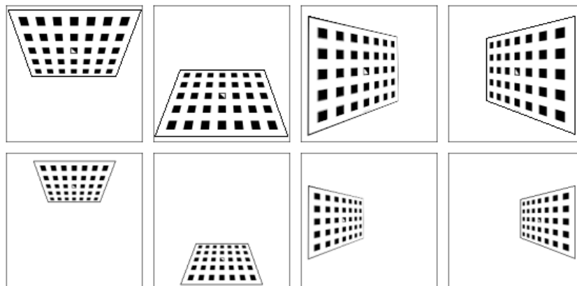
Abb. 5.23: Empfohlene Ansichten des Kalibriermusters während des Kalibriervorgangs. Im Fall von 4DOF-Robotern müssen andere Ansichten gewählt werden, welche so unterschiedlich wie möglich sein sollten.
