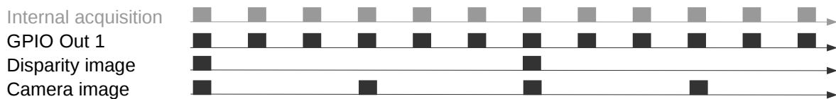
Abb. 5.35: Beispiel für die Nutzung der Betriebsart ExposureActive für GPIO-Ausgang 1 mit einer benutzerdefinierten Bildwiederholrate von 8 Hz. Die interne Bildaufnahme geschieht immer mit 25 Hz. GPIO-Ausgang 1 ist für die Dauer der Belichtungszeit jedes Bildes an (HIGH). Disparitätsbilder werden für Kamerabilder berechnet, die auch per GigE Vision in der benutzerdefinierten Bildwiederholrate versendet werden.
