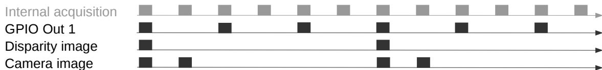
Abb. 5.36: Beispiel für die Nutzung der Betriebsart ExposureAlternateActive für GPIO-Ausgang 1 mit einer benutzerdefinierten Bildwiederholrate von 8 Hz. Die interne Bildaufnahme geschieht immer mit 25 Hz. GPIO-Ausgang 1 ist für die Dauer der Belichtungszeit jedes zweiten Bildes an (HIGH). Disparitätsbilder werden für Kamerabilder berechnet, bei denen GPIO-Ausgang 1 an (HIGH) ist, und die auch per GigE Vision in der benutzerdefinierten Bildwiederholrate versendet werden. In der Betriebsart ExposureAlternateActive werden Intensitätsbilder immer paarweise versendet: ein Bild mit GPIO-Ausgang 1 an (HIGH), für das ein Disparitätsbild verfügbar sein kann, und ein Bild mit GPIO-Ausgang 1 aus (LOW).
