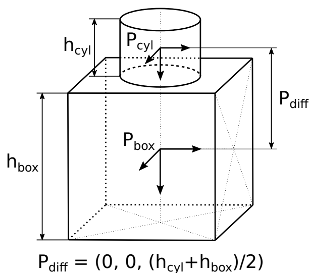
Abb. 6.42: Bezugskoordinatensysteme für das Erstellen von Greifern über die REST-API und die Web GUI
