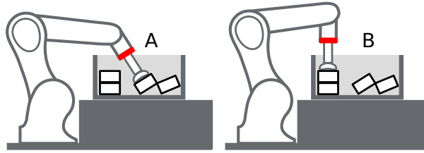
Abb. 6.41: Fall A: Der Griff wird nur als Kollision erkannt, wenn check_flange auf true gesetzt ist, denn der Flansch (rot) befindet sich im Load Carrier. Fall B: Der Griff ist in jedem Fall kollisionsfrei.
